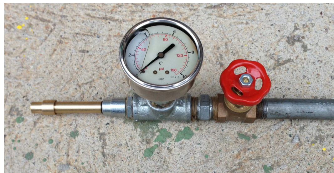
UGELLO CON SUPPORTO, MANOMETRO E VALVOLA A SARACINESCA
