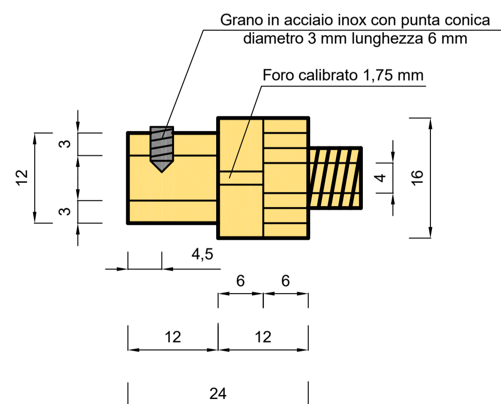
SEZIONE UGELLO
